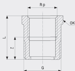
Redukcija - bronca Model 3244
