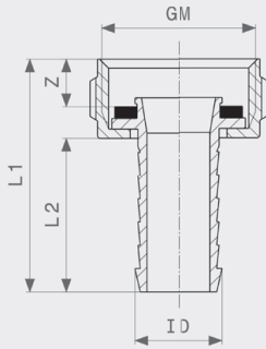
Navojna spojnica za crijevo - mesing Model 1817
