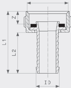
Navojna spojnica za crijevo - mesing Model 1819
