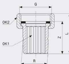
Priključna navojna spojnica - bronca Model 3335
