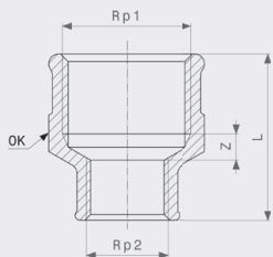
Reducir spojnica - bronca Model 3240
