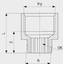
Redukcija - bronca Model 3242
