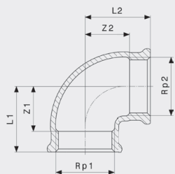
Koljeno 90° - bronca Model 3090
