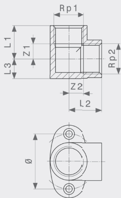
Zidna pločica - mesing Model 1421
