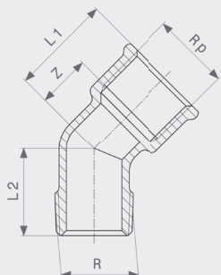
Koljeno 45° - mesing Model 1615
