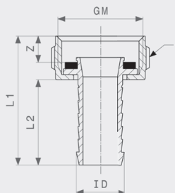
Navojna spojnica za crijevo - mesing Model 1814
