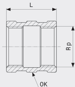
Spojnica - bronca Model 3270
