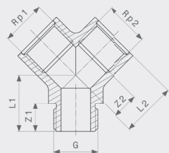
Dvostruki priključni komad - mesing Model 1641
