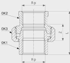
Navojna spojnica - bronca Model 3340
