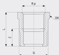
Redukcija - bronca Model 3244
