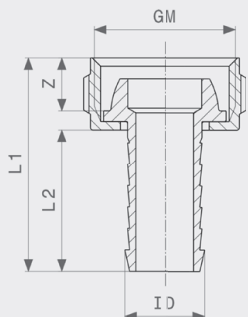
Navojna spojnica za crijevo - mesing Model 1812
