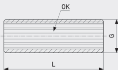
Dugačka spojnica - bronca Model 3535
