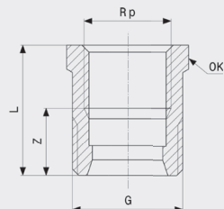
Redukcija - bronca Model 3243
