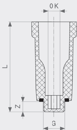
Čep za tlačnu probu - umjetni materijal Model 1516
