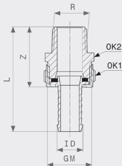
Navojna spojnica za krutu cijev - mesing Model 1831
