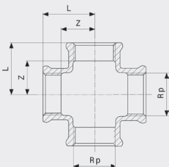
Križni komad - bronca Model 3180
