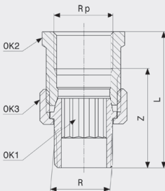
Navojna spojnica - bronca Model 3341
