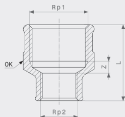
Reducir spojnicica - bronca Model 3240
