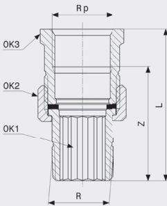
Navojna spojnica - bronca Model 3331
