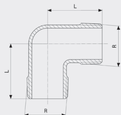
Koljeno 90° - bronca Model 3091
