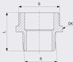
Redukcija - bronca Model 3247
