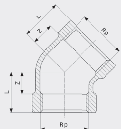
Koljeno 45° - bronca Model 3120
