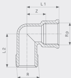
Koljeno 90° - mesing Model 1613
