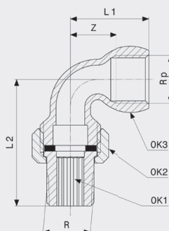
Navojna spojnica - bronca Model 3088
