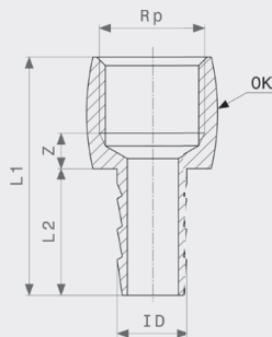
Tuljak za crijevo - mesing Model 1846
