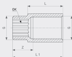
Produžetak za slavinu - bronca Model 3526
