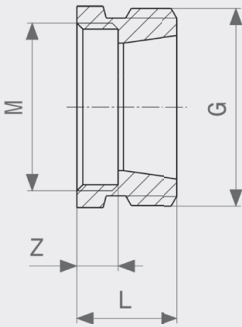
Redukcija - bronca Model 3251
