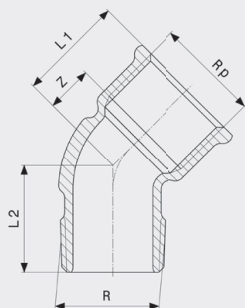
Koljeno 45° - bronca Model 3121
