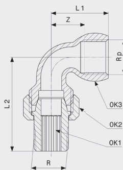
Navojna spojnica - bronca Model 3098
