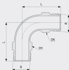
Koljeno 90° - bronca Model 3003
