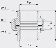
Navojna spojnica - bronca Model 3330
