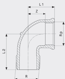
Koljeno 90° - bronca Model 3092
