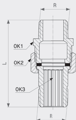
Navojna spojnica - bronca Model 3334
