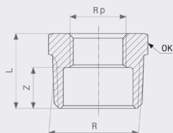
Redukcija - bronca Model 3241
