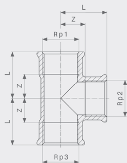
T-komad - mesing Model 1622
