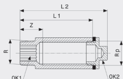
Produžetak za slavinu - bronca Model 3527
