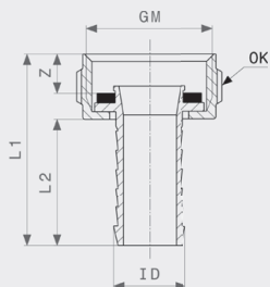
Navojna spojnica za crijevo - mesing Model 1811
