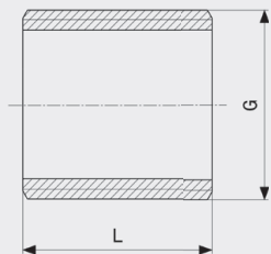
Spojnica - bronca Model 3531
