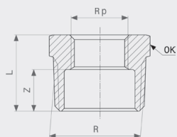
Redukcija - bronca Model 3241
