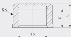
Kapa - bronca Model 3301
