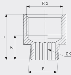
Redukcija - bronca Model 3242
