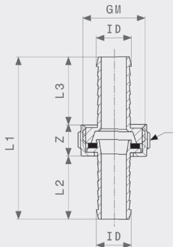
Navojna spojnica za crijevo - mesing Model 1821
