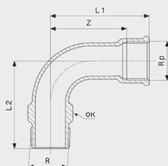
Koljeno 90° - bronca Model 3001
