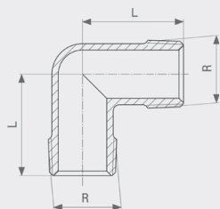
Koljeno 90° - mesing Model 1611
