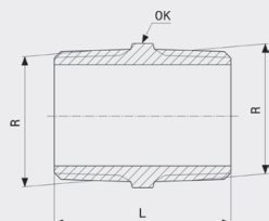
Dvostruka spojnicica - bronca Model 3280
