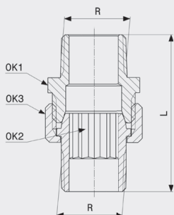
Navojna spojnica - bronca Model 3344
