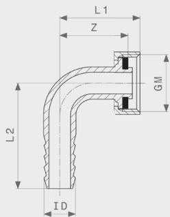
Navojna spojnica za crijevo - mesing Model 1813
