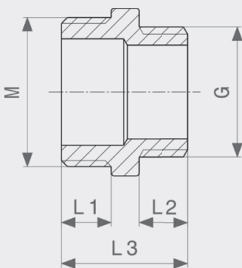
Redukcija - bronca Model 3253
