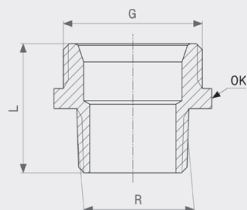
Redukcija - bronca Model 3246
