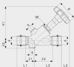
Easytop Inox-KRV kosi nasjedni ventil - nehrđajući čelik Model 2338
