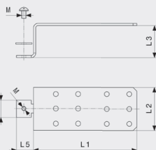
Držač - pocinčani čelik Model 2141.4
