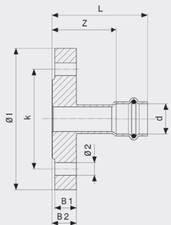
Sanpress Inox-Prirubnički prijelaz - nehrđajući čelik Model 2359
