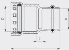
Megapress-Prijelazni komad - silicijeva bronca Model 4213.2
