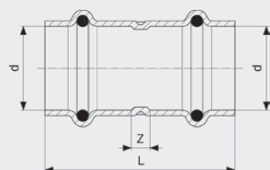
Sanpress Inox-Spojnicica - nehrđajući čelik Model 2315
