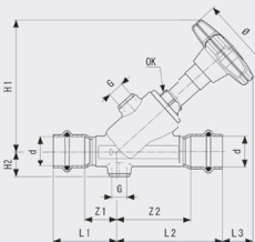
Easytop Inox-KRV kosi nasjedni ventil - nehrđajući čelik Model 2338.5
