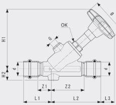
Easytop Inox-Kosi nasjedni ventil - nehrđajući čelik Model 2337.5
