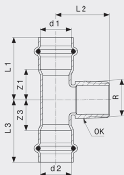
Sanpress Inox-T-komad - nehrđajući čelik Model 2317.1
