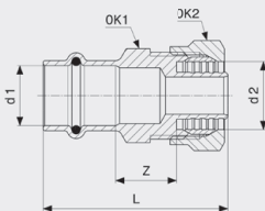
Sanpress-Prijelazna navojna spojnica - bronca Model 2213
