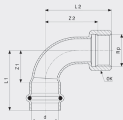
Sanpress Inox-Prijelazno koljeno 90° - nehrđajući čelik Model 2314.5
