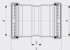
Sanpress Inox XL-Spojnicica - nehrđajući čelik Model 2315XL
