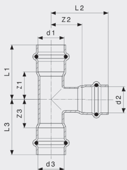
Sanpress Inox-T-komad - nehrđajući čelik Model 2318
