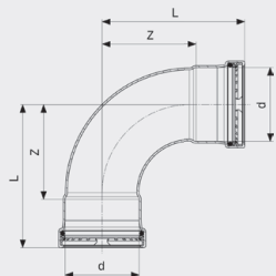
Sanpress Inox XL-Koljeno 90° - nehrđajući čelik Model 2316XL
