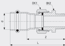
Sanpress Inox-Prijelazna navojna spojnica - nehrđajući čelik Model 2365
