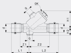
Easytop Inox-Ventil s nepovratnom zaklopom - nehrđajući čelik Model 2339.4
