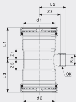
Sanpress Inox-T-komad - nehrđajući čelik Model 2317.2
