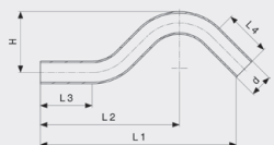
Sanpress-Nadvoj - nehrđajući čelik Model 2209.3
