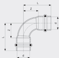
Sanpress Inox-Koljeno 90° - nehrđajući čelik Model 2316
