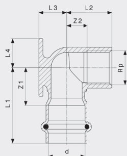
Sanpress Inox-Zidna pločica - nehrđajući čelik Model 2325.5
