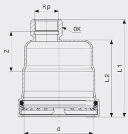
Sanpress Inox XL-Kapa - nehrđajući čelik Model 2356XL
