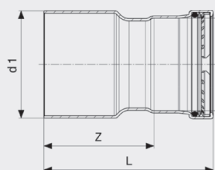
Sanpress Inox XL-Redukcija - nehrđajući čelik Model 2315.1XL
