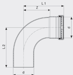
Sanpress Inox XL-Koljeno 90° - nehrđajući čelik Model 2316.1XL
