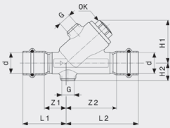
Easytop Inox-Ventil s nepovratnom zaklopkom - nehrđajući čelik Model 2339
