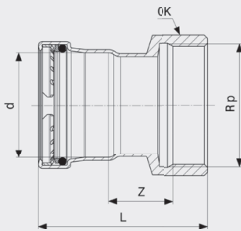
Sanpress Inox-Prijelazni komad - nehrđajući čelik Model 2312
