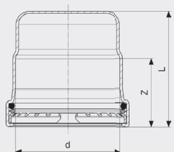
Sanpress Inox XL-Kapa - nehrđajući čelik Model 2356.1XL
