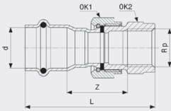
Sanpress Inox-Prijelazna navojna spojnica - nehrđajući čelik Model 2362
