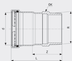
Sanpress Inox-Prijelazni komad - nehrđajući čelik Model 2311
