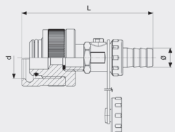
Čep za tlačnu probu - mesing Model 2269
