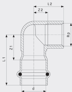
Sanpress Inox-Prijelazni luk 90° - nehrđajući čelik Model 2314.2
