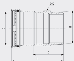
Sanpress Inox XL-Prijelazni komad - nehrđajući čelik Model 2311XL
