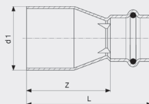
Sanpress Inox-Redukcija - nehrđajući čelik Model 2315.1
