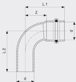
Sanpress Inox-Koljeno 90° - nehrđajući čelik Model 2316.1
