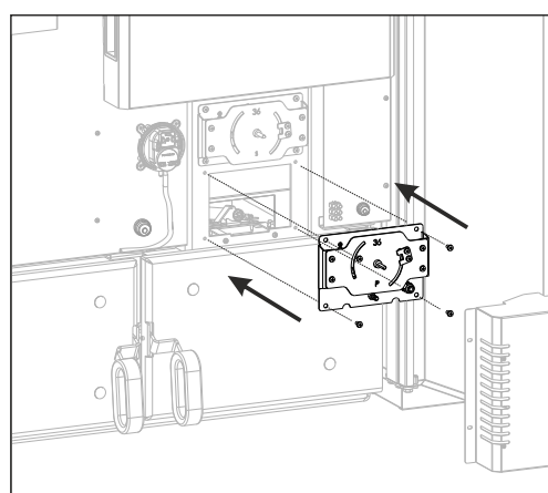
Detalj B
