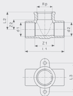
Zidna pločica s T-komadom - bronca Model 94490G
