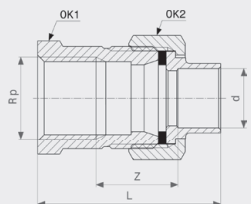
Prijelazna navojna spojnica - bronca, mesing Model 94330G
