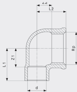
Prijelazni luk 90° - bronca Model 94090G
