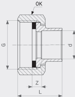
Priključna navojna spojnica Model 94359
