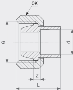
Priključna navojna spojnica - bronca Model 94384G
