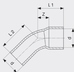
Koljeno 45° - bakar Model 95040
