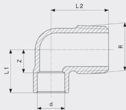
Prijelazni luk 90° - bronca Model 94092G
