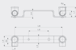
Gemini-Montažna jedinica Model 94476.1
