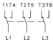
HEMA SPAJANJA
