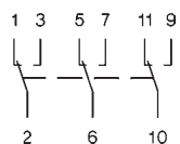
HEMA SPAJANJA
