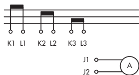
HEMA SPAJANJA
