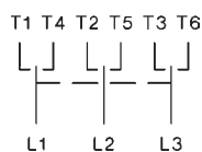
HEMA SPAJANJA
