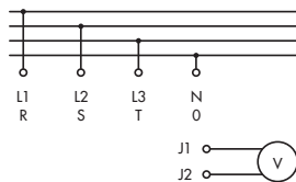
HEMA SPAJANJA
