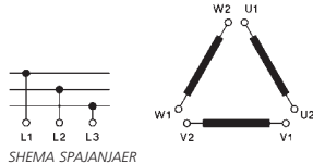
HEMA SPAJANJAER
