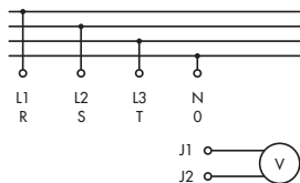
HEMA SPAJANJA
