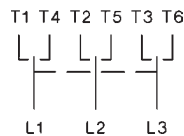
HEMA SPAJANJA
