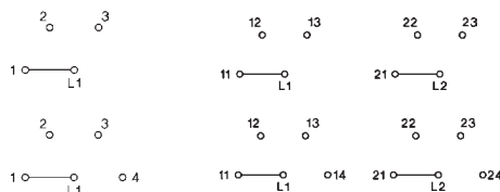
HEMA SPAJANJA 1-polna
