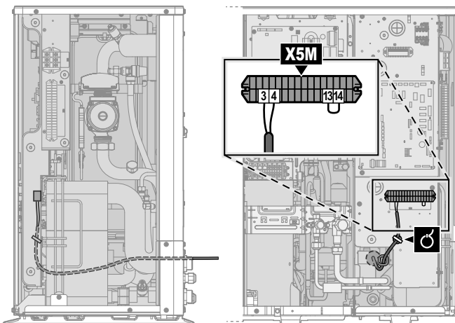
S4S Smart Grid strujomjer
