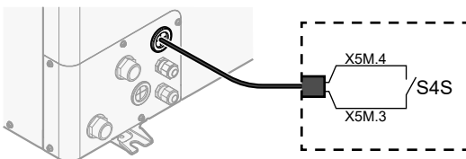
S4S Smart Grid strujomjer
