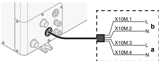
a, b Smart Grid visokonaponski kontakti
