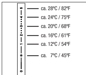
Abb.5 Temperaturskala Thermostat „vindo TH“
