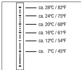
Obr.5 Teplotní stupnice termostatické hlavice „vindo TH“
