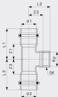
Prestabo-T-komad - nelegirani pocinčani čelik Model 1117.2
