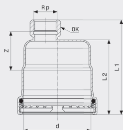
Prestabo XL-Kapa - nelegirani pocinčani čelik Model 1156XL
