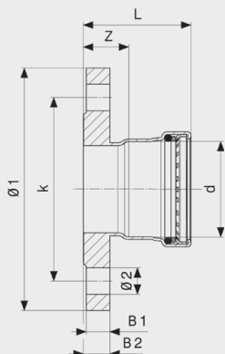
Prestabo XL-Prirubnički prijelaz - nelegirani pocinčani čelik Model 1159.1XL
