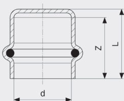
Prestabo-Kapa - nelegirani pocinčani čelik Model 1156
