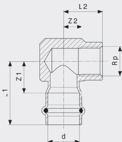
Prestabo-Prijelazni luk 90° - nelegirani pocinčani čelik Model 1114.2
