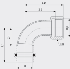
Prestabo-Prijelazno koljeno 90° - nelegirani pocinčani čelik Model 1114.5
