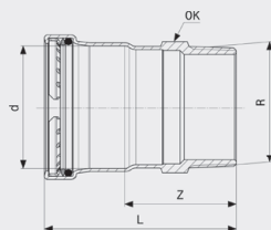
Prestabo-Prijelazni komad - nelegirani pocinčani čelik Model 1111
