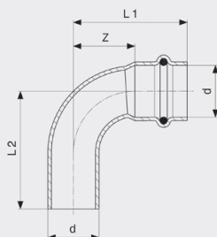
Prestabo-Koljeno 90° - nelegirani pocinčani čelik Model 1116.1
