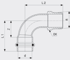
Prestabo-Prijelazno koljeno 90° - nelegirani pocinčani čelik Model 1114
