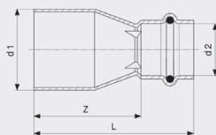
Prestabo-Redukcija - nelegirani pocinčani čelik Model 1115.1
