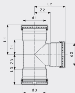
Prestabo XL-T-komad - nelegirani pocinčani čelik Model 1118XL
