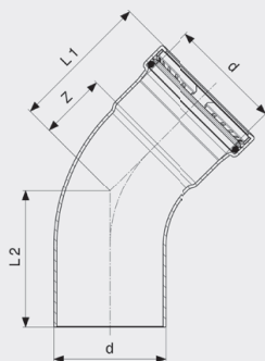
Prestabo XL-Koljeno 45° - nelegirani pocinčani čelik Model 1126.1XL
