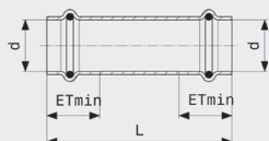
Prestabo-Klizna spojnicca - nelegirani pocinčani čelik Model 1115.5
