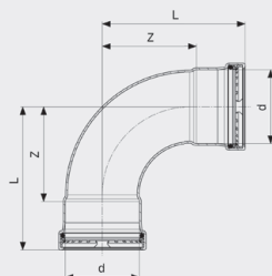
Prestabo XL-Koljeno 90° - nelegirani pocinčani čelik Model 1116XL
