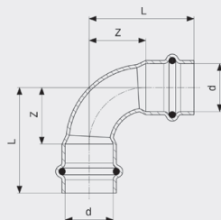
Prestabo-Koljeno 90° - nelegirani pocinčani čelik Model 1116
