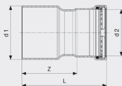
Prestabo XL-Redukcija - nelegirani pocinčani čelik Model 1115.1XL
