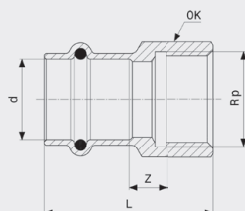
Prestabo-Prijelazni komad - nelegirani pocinčani čelik Model 1112
