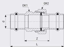
Prestabo-Navojna spojnica - nelegirani pocinčani čelik Model 1160
