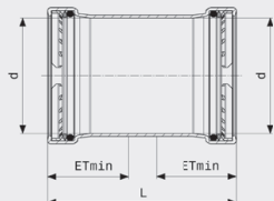
Prestabo XL-Klizna spojnicca - nelegirani pocinčani čelik Model 1115.5XL
