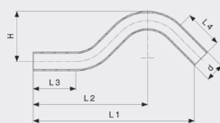
Prestabo-Nadvoj - nelegirani pocinčani čelik Model 1109.3
