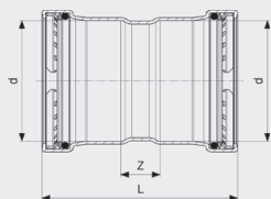
Prestabo XL-Spojnicca - nelegirani pocinčani čelik Model 1115XL
