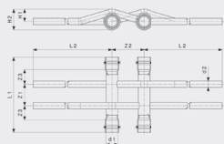
Prestabo-Razdjeljivač ogranaka Model 1149.7
