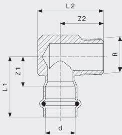
Prestabo-Prijelazni luk 90° - nelegirani pocinčani čelik Model 1114.1
